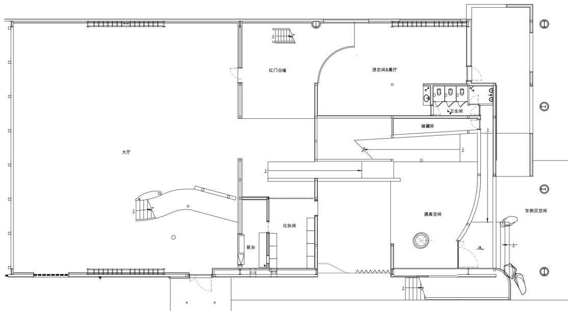
一层平面图 900平
