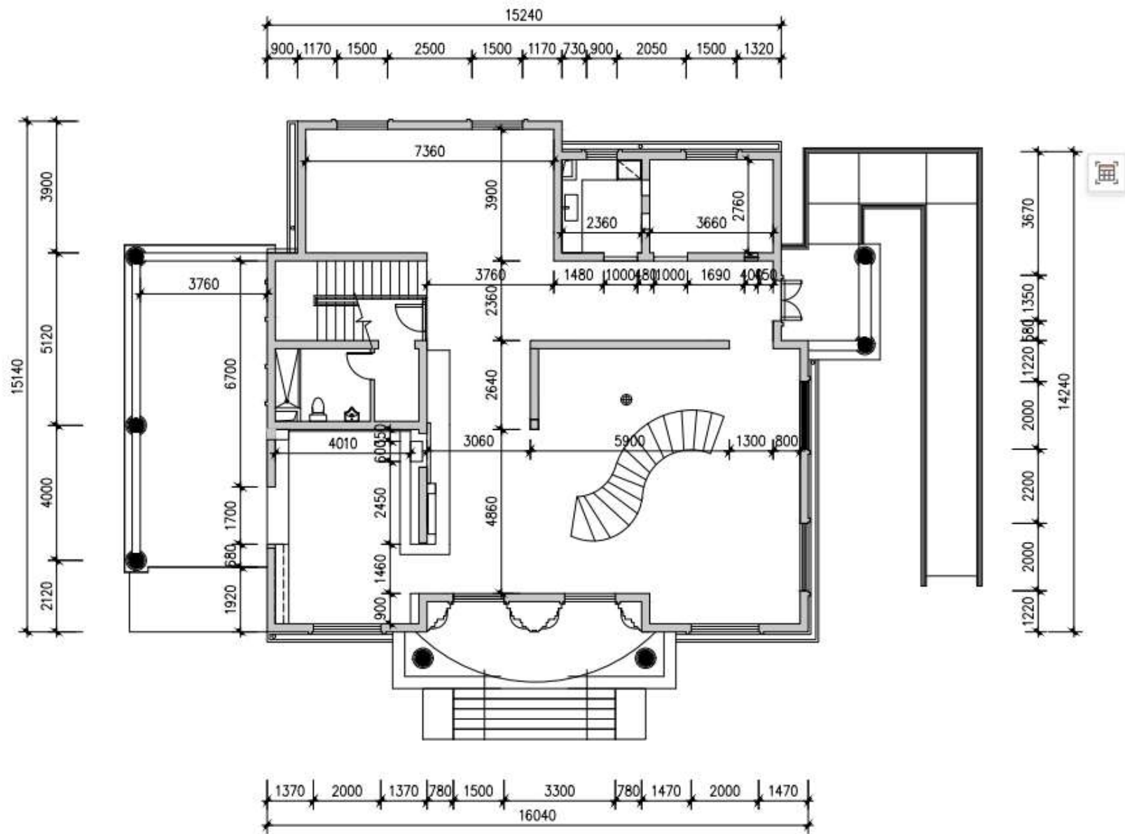
一层平面布置图
